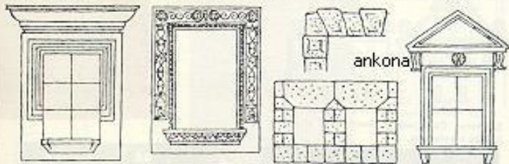
Český Krumlov (kolem r. 1520) - pro renesanci typické pravoúhlé zalomení celého profilu ve výši "soklu", Pardubice (po r. 1538) - sériově pálené keramické ostění s rozvilinami, erby a motivy kandelábrů, bosová ostění (šambrány), Chrudim čp. 5 (1573) - okno s trojúhelníkovým frontonem na konzolách - zvaných ankona
